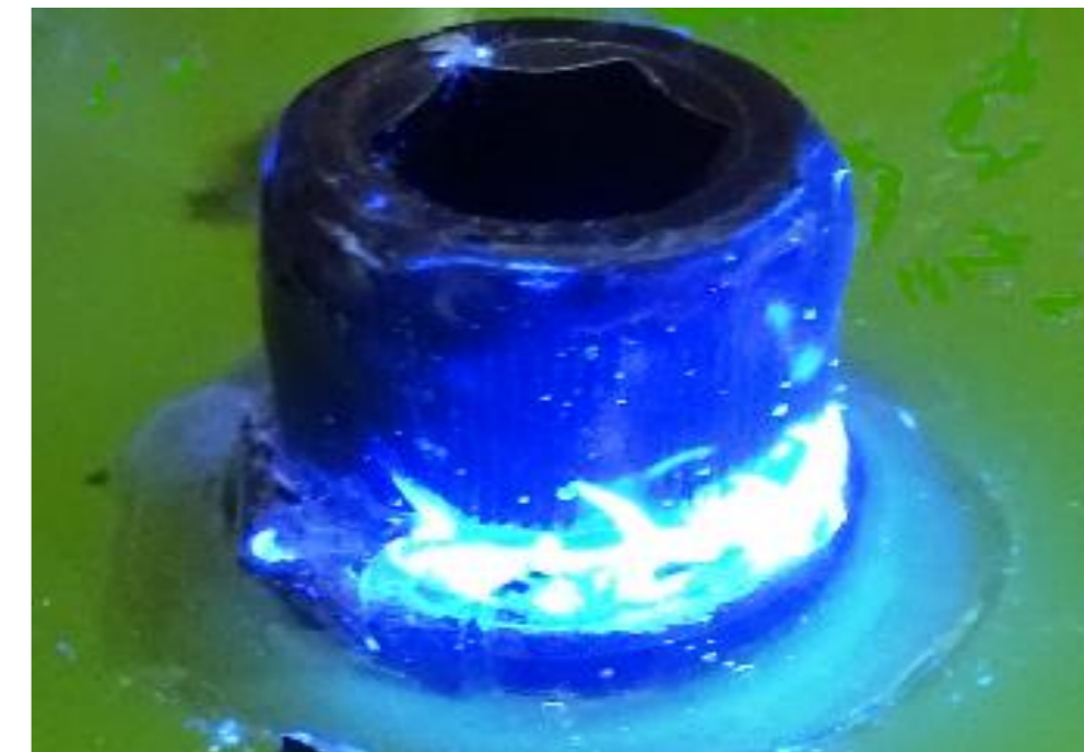
紫外線照射によるネジの緩みの発光状況
