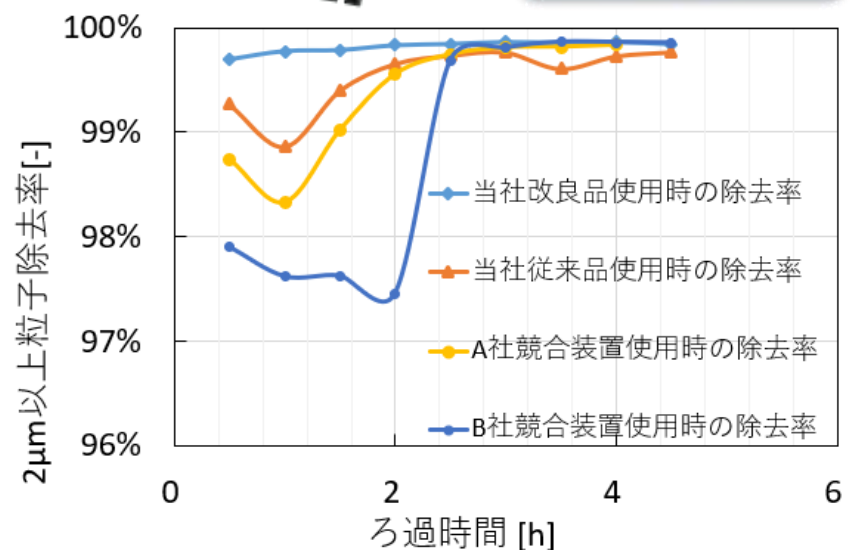
図1 関東ローム添加した模擬液のろ過試験
